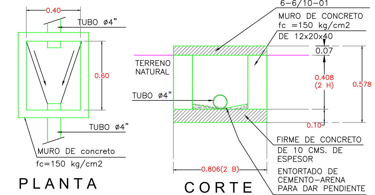
DETALLE DE REGISTRO SANITARIO S/ESC.
